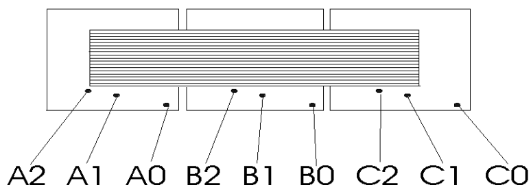
Trafo ATP 60.2- značení vývodů (pohled zvrchu)
