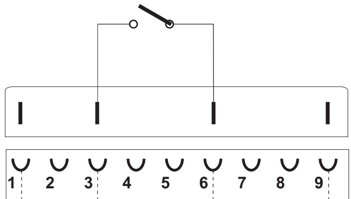
Centrální konektor hořáku Torch central connector
