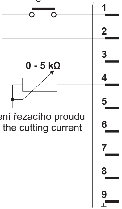
Konektor dálkového ovládání Remote ctrl connector
