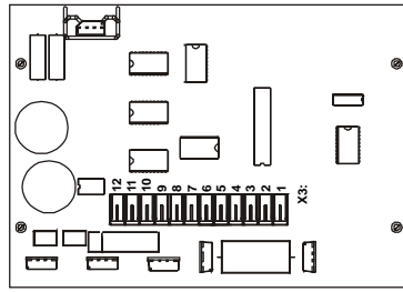
ČÍSLOVÁNÍ SVOREK PCB DC1.0 (POHLED ZE ZADNÍ STRANY)
