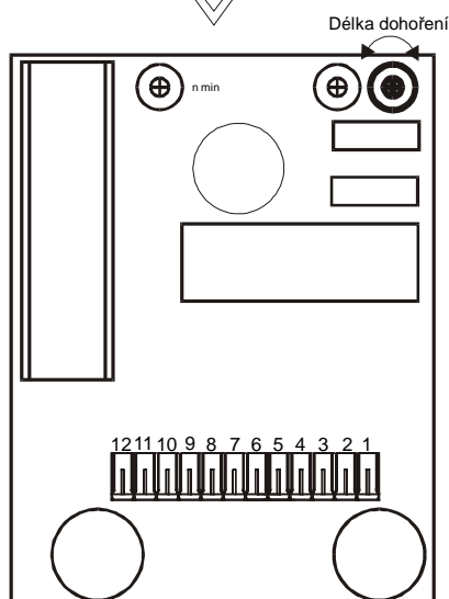
2802 PCB D22V3.1
