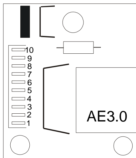
2484 PCB AE3.0
