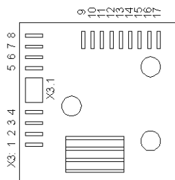
Číslování svorek (pohled ze zadu)
