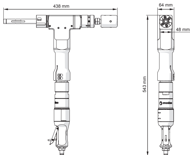
PRO-2 PB s pneumatickým pohonem
