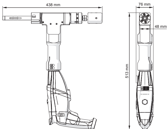
PRO-2 PB s elektrickým motorem
