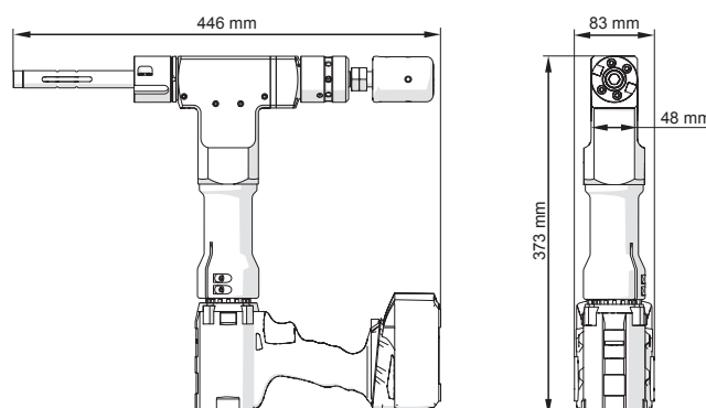
PRO-2 PB s aku pohonem
