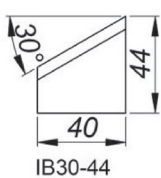
30° Nástrojový nůž pro vnitřní obrábění, Výška 44 mm [IB30/44] Číslo produktu: NOZ-000023
