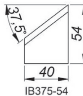
37.5° Nástrojový nůž pro vnitřní obrábění, Výška 54 mm [IB375/54] Číslo produktu: NOZ-000024
