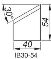
30° Nástrojový nůž pro vnitřní obrábění, Výška 54 mm [IB30/54] Číslo produktu: NOZ-000025
