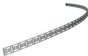
Flexibilní vodící lišta - délka 185cm (6ft) 1ks Minimální poloměr zakřivení 1,0 m (3,3 ft) PRW-0466-50-01-01-0
