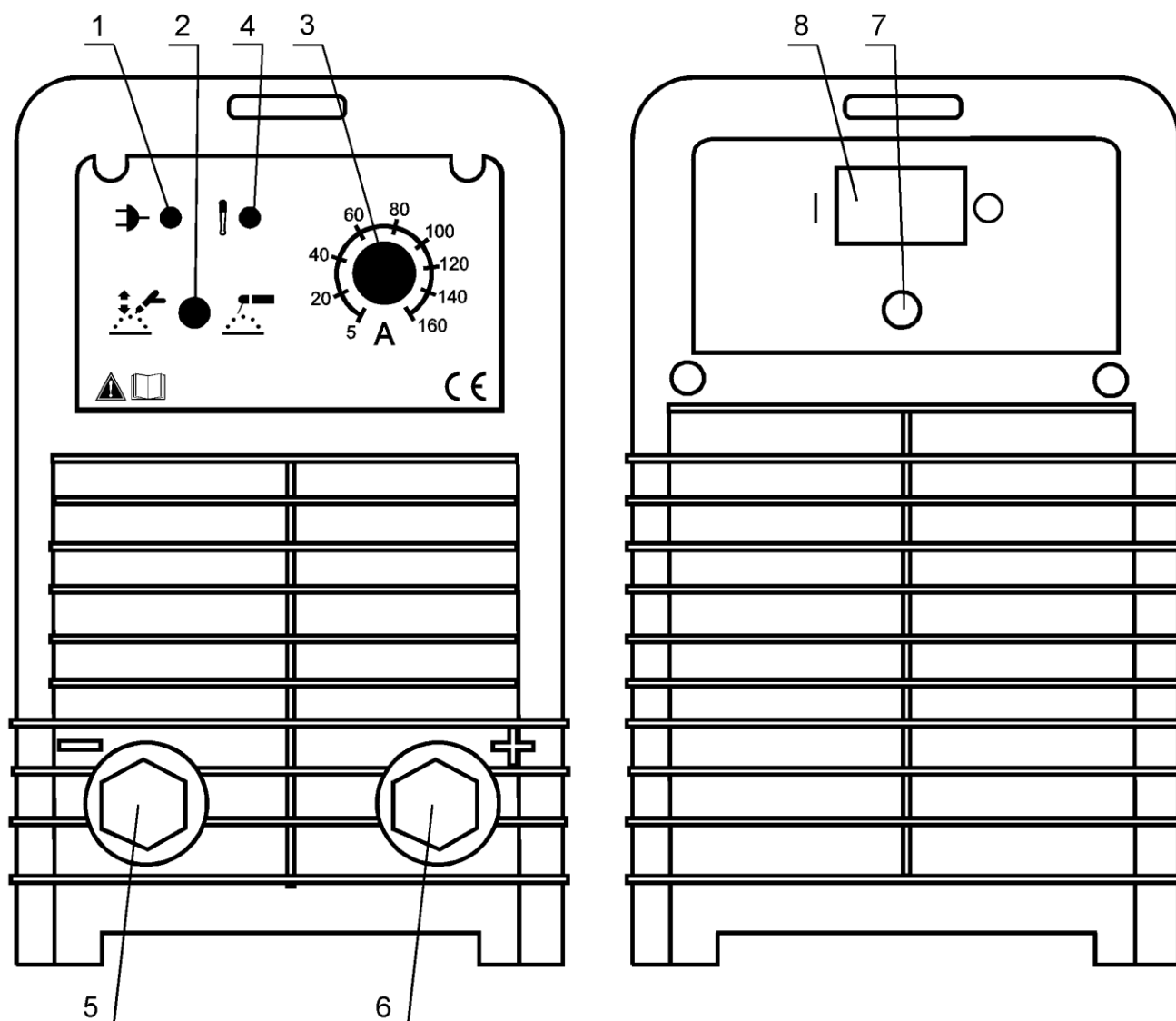
FIG. 1- Parti generali della macchina
